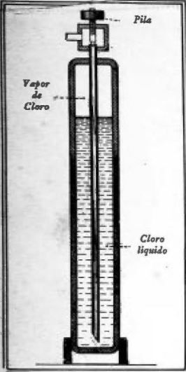
Corte de la botella proyectora de gases.
